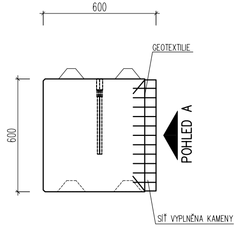
ŘEZ 1-1
