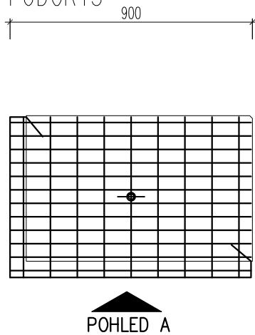
PŮDORYS
